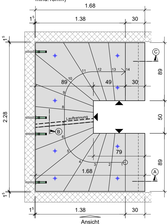
GRUNDRISS (Fugen zum Rohbau mind. 15mm)
