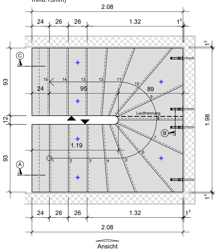
GRUNDRISS (Fugen zum Rohbau mind.15mm)
