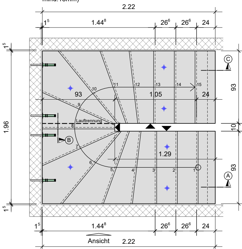
GRUNDRISS
