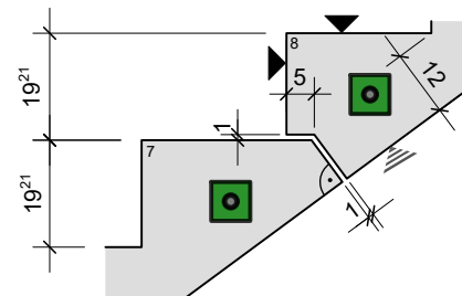
DETAIL B Lauftrennung
