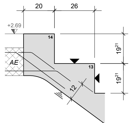
DETAIL B Lauftrennung
