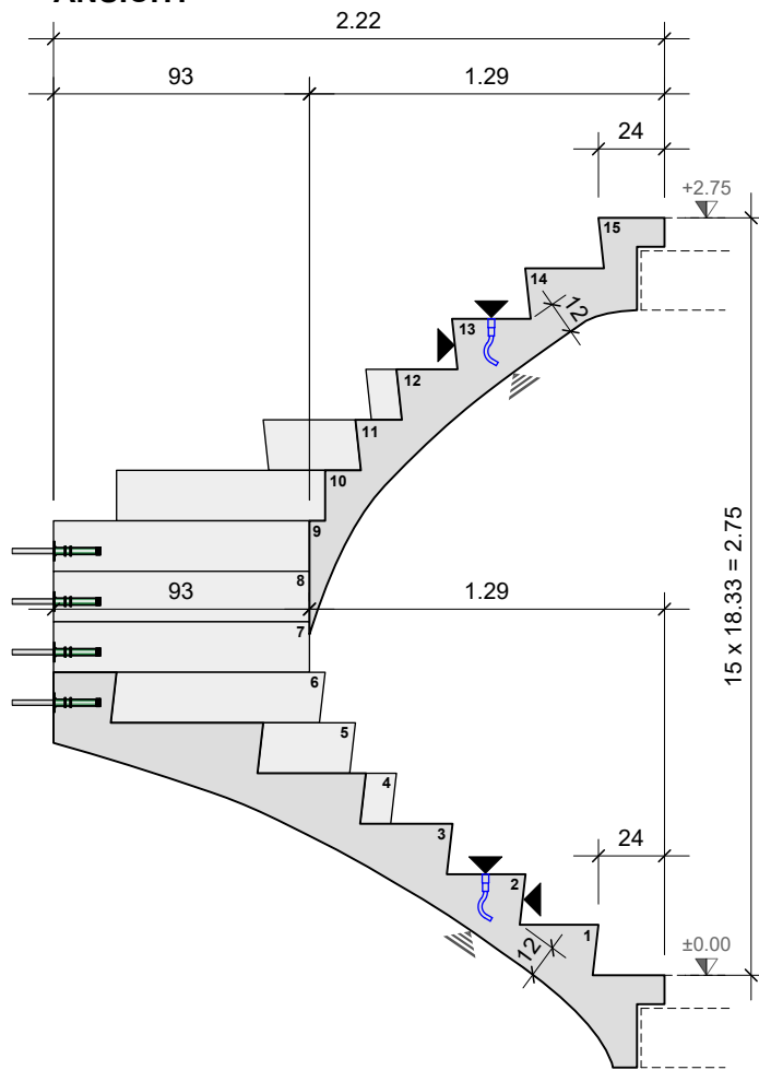
ANSICHT
