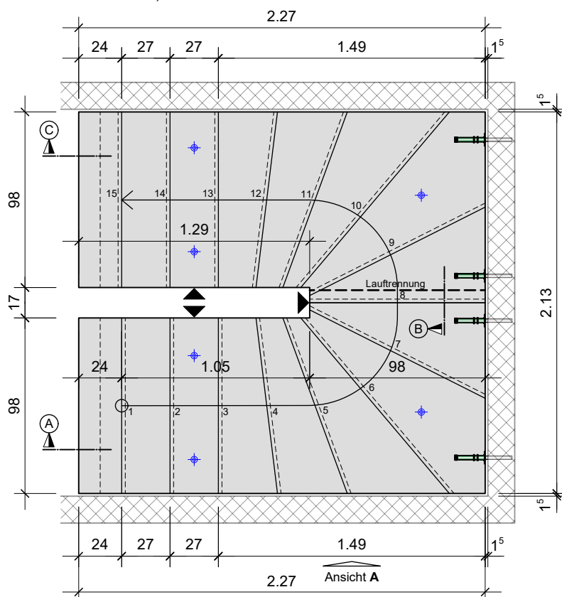
GRUNDRISS (Fugen zum Rohbau mind.15mm)
