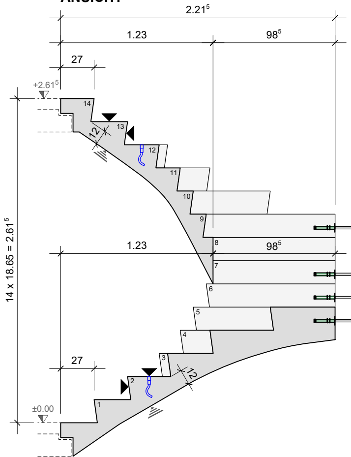
ANSICHT
