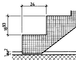
SCHNITT UG
