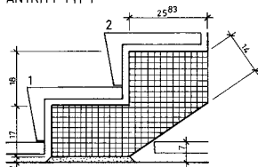
ANTRITT TYP 1A
