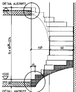
SCHNITT A-A
