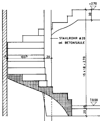
SCHNITT D-D
