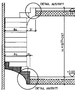
SCHNITT A-A
