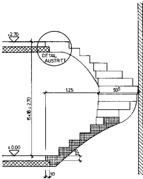
SCHNITT A-A
