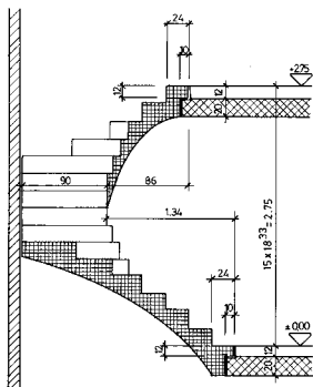
SCHNITT A-A
