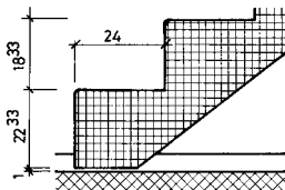
SCHNITT UG-EG
