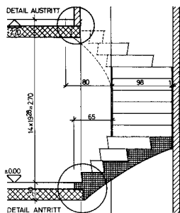
SCHNITT A-A
