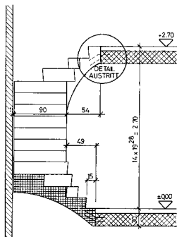
SCHNITT A-A
