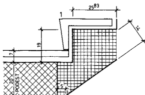
ANTRITT TYP 1
