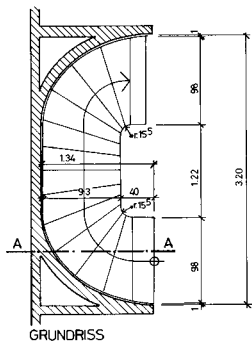
GRUNDRISS
