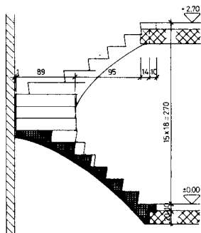
SCHNITT A-A
