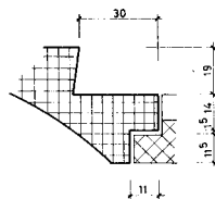
Schnitt B-B
