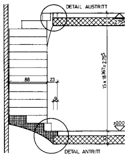
SCHNITT A-A
