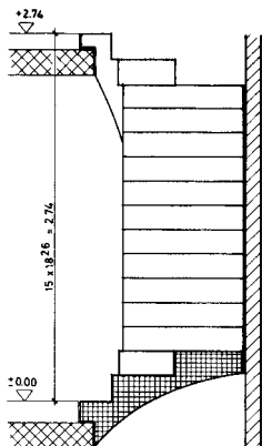
SCHNITT A-A
