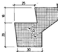
DETAIL AUSTRITT IM UG
