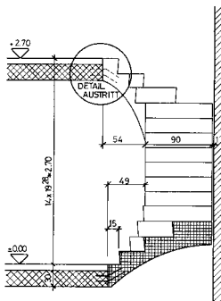
SCHNITT A-A
