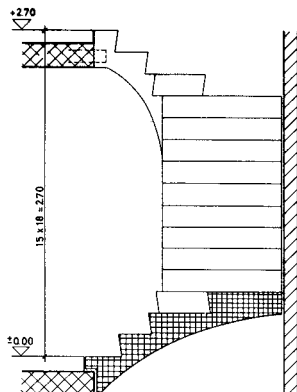
SCHNITT A-A
