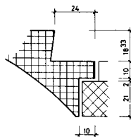
SCHNITT B-B
