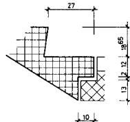
SCHNITT B-B
