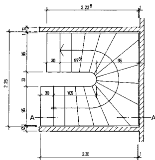
GRUNDRISS
