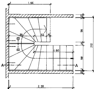
GRUNDRISS
