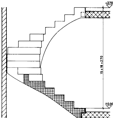
SCHNITT A - A
