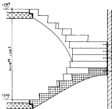
SCHNITT A-A
