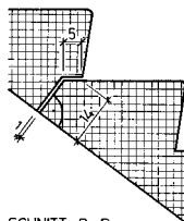
SCHNITT B-B
