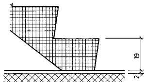
DETAIL AUSTRITT IM UG
