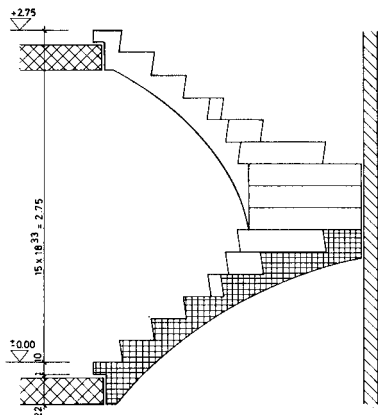
SCHNITT A-A
