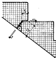
SCHNITT B-B
