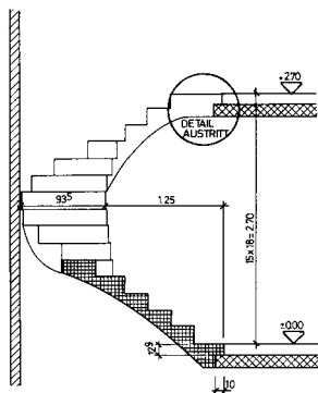
SCHNITT A-A
