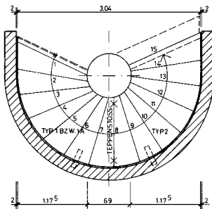
ANTRITT TYP 1A
