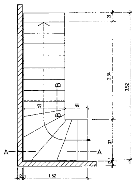
GRUNDRIS
