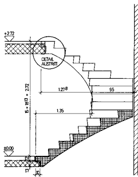
SCHNITT A-A
