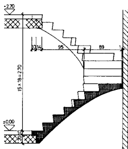
SCHNITT A-A
