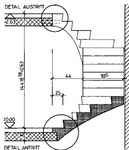
SCHNITT A-A
