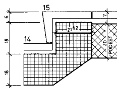
AUSTRITT TYP 2
