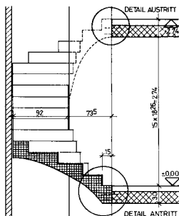
SCHNITT A-A
