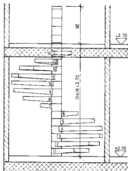
ANSICHT
