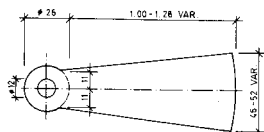
GRUNDRISS
