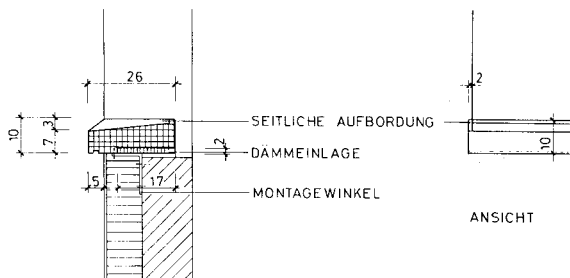
FENSTERBANK MIT DÄMMEINLAGE UND SEITLICHER AUFBORDUNG
