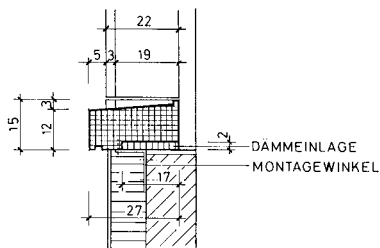
FENSTERBANK MIT DÄMMEINLAGE
