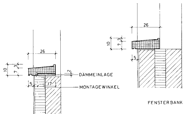
FENSTERBANK MIT DÄMMEINLAGE UND SEITLICHER AUFBORDUNG
